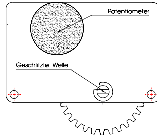
Abb.4: Potentiometer mit Fernsendergetriebe
