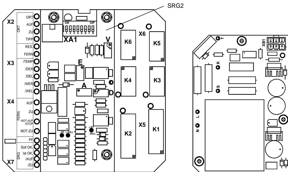
Abb.1: Logikplatine mit Stellungsregler SRG
