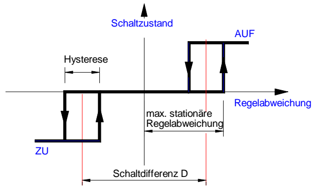
Abb.5: Schaltpunkte des 3-Punktreglers
